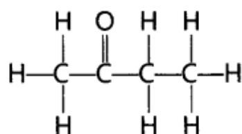
Butanone
